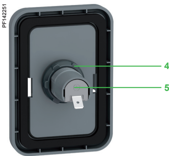
用于在机箱门上安装基本中文面板的远程安装套件(后面)
