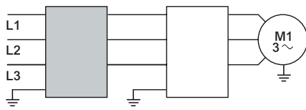
附加EMC 滤波器 带有集成式滤波器的 ATV340●●●N4 ATV340●●●N4E
