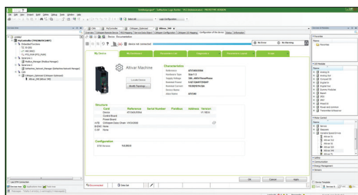
SoMachine中的ATV340DTM
