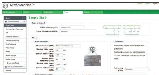
驱动参数标签页
